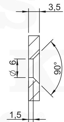
SEZIONE B-B
