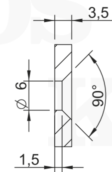
SEZIONE C-C
